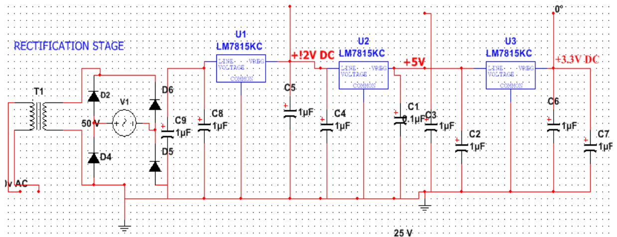
Fig 5.4.3 (4) Rectification Circuit-D
