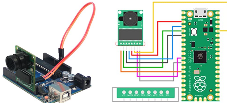
Figure 30 Arducam Mini Module OV2640
