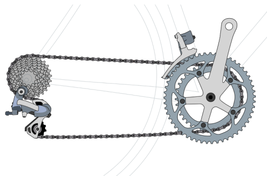
Figure 2. Derailleur System
