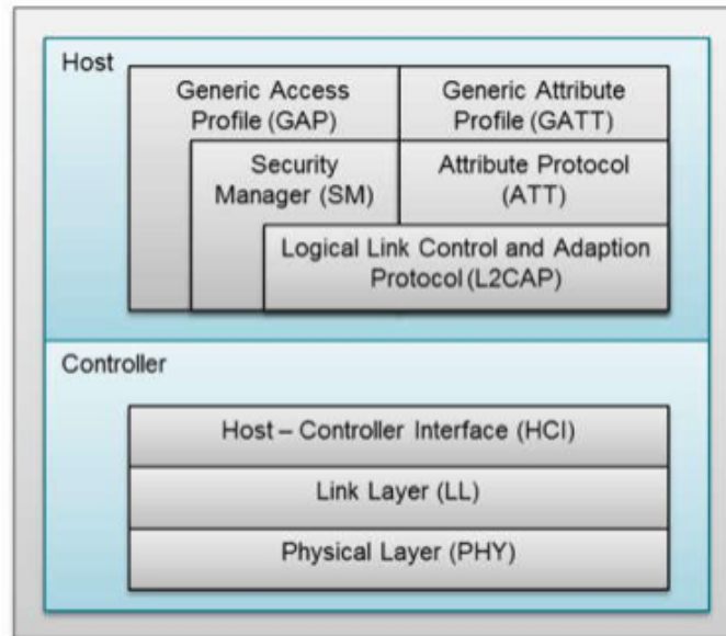
Figure 44. The BLE protocol stack
